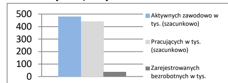
Rejestr bezrobotnych
