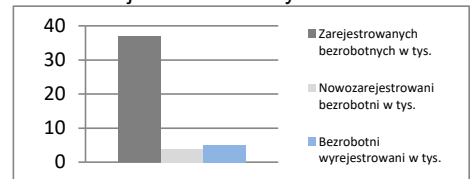
Dynamiki - przemysł
