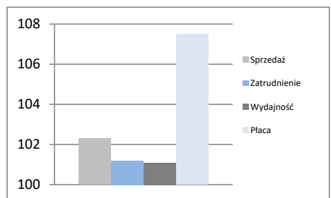
Dynamiki - budownictwo
