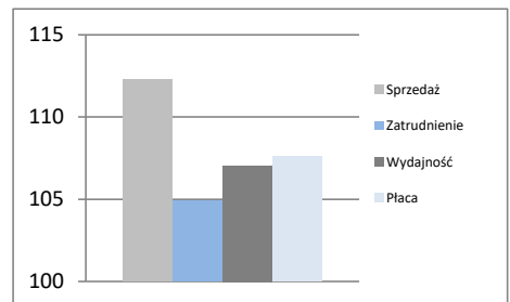
Dynamiki - budownictwo
