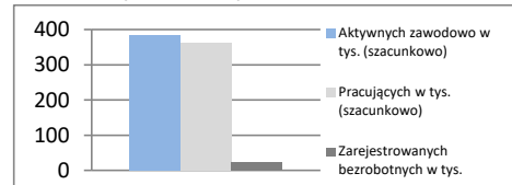
Rejestr bezrobotnych
